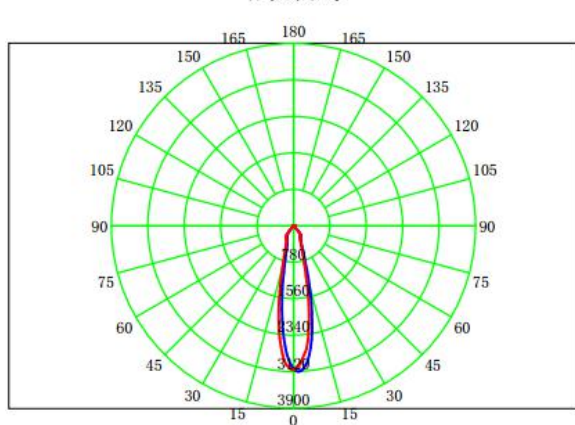
配光曲线
